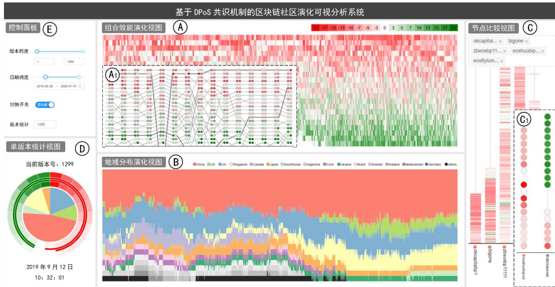
图 1 基于 DPoS 共识机制的区块链社区演化可视分析系统
